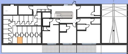
Übersicht Erdgeschoss / Lagerbereich
